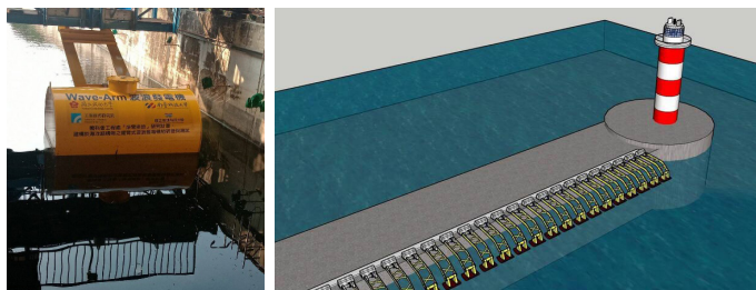
「擎浪者」波浪發電機（左）及此機組安裝於防波堤的預想圖（右）。
